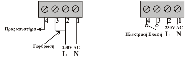
Διάγραμμα Συνδεσμολογίας
