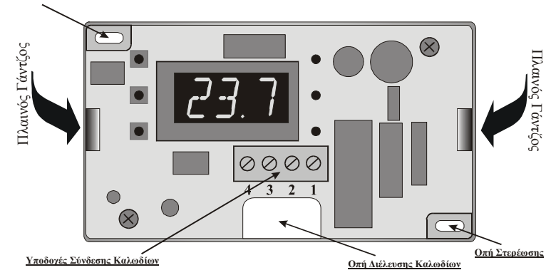
Παράδειγμα για καυστήρες 230V
